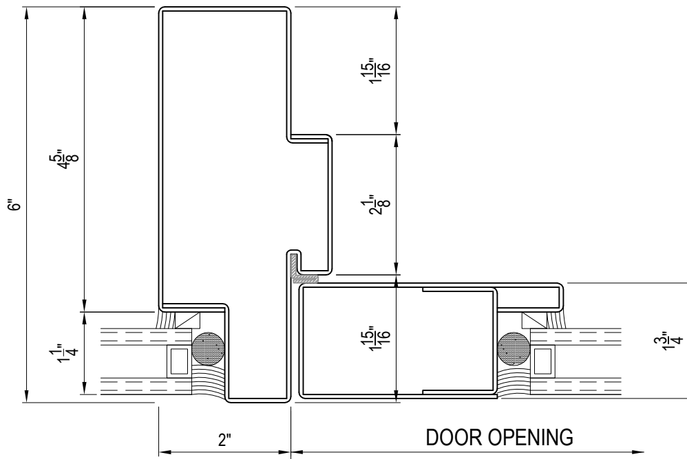
DOOR JAMB
