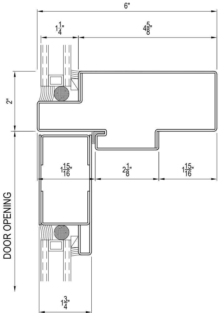
DOOR HEADER
